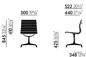
EA 101, nicht drehbar, ohne Armlehnen
