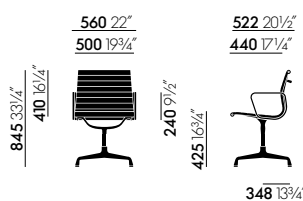
EA 103, nicht drehbar, mit Armlehnen
